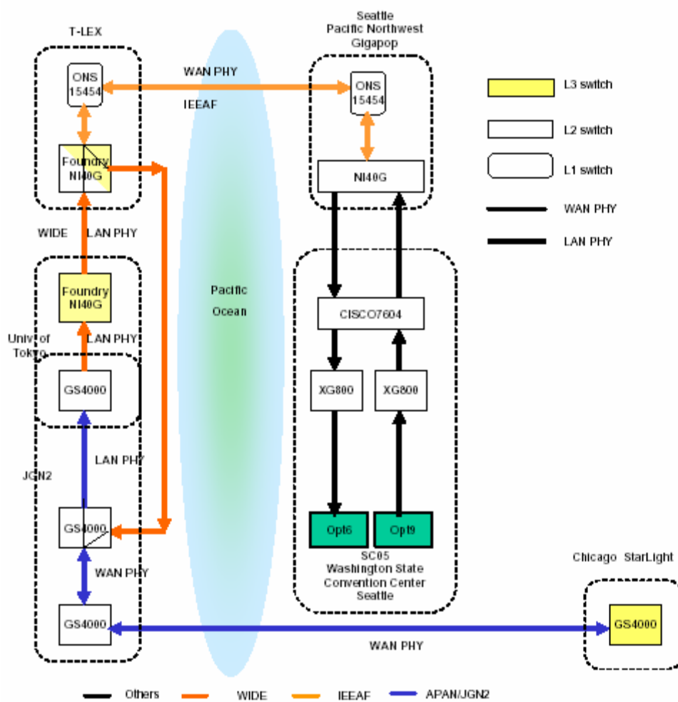
ネットワーク経路、ルータ、スイッチの詳細 (IPv6)
