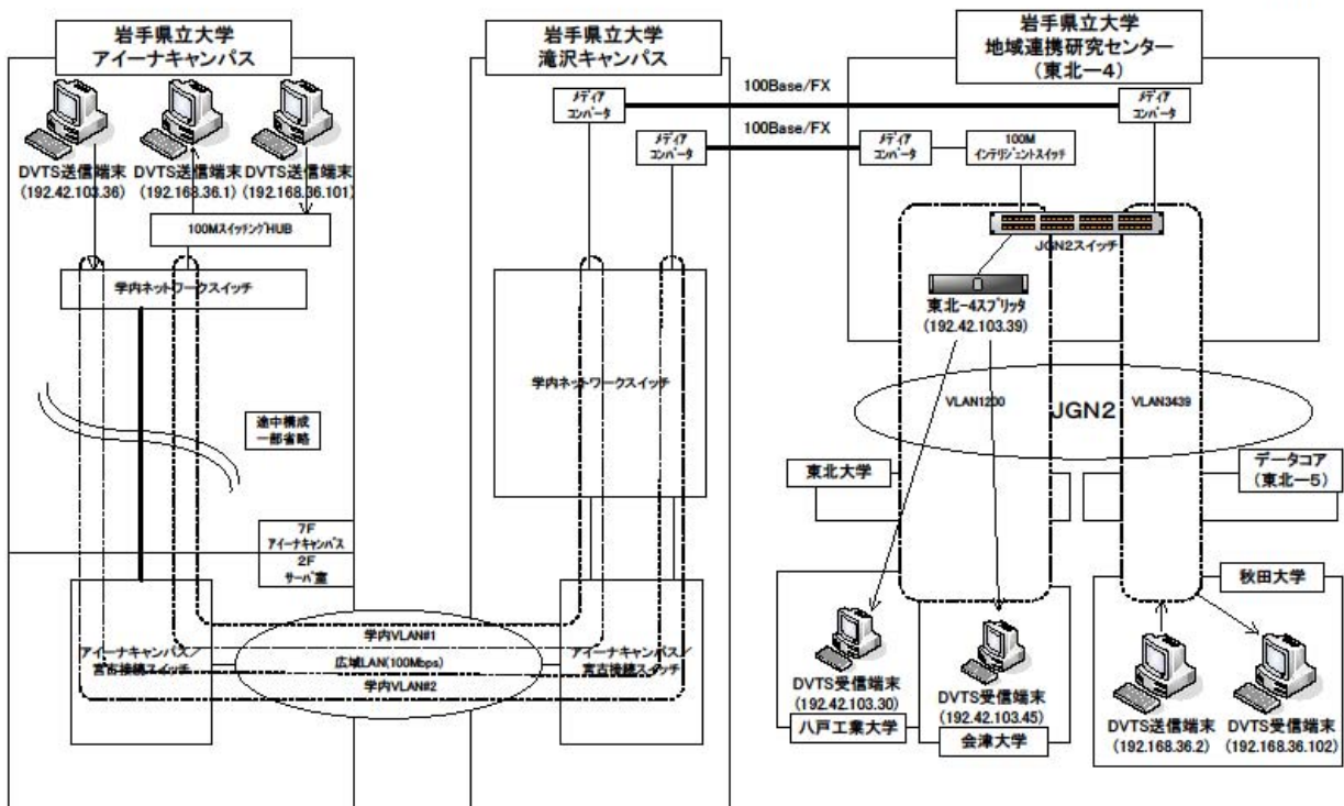
2007/3/6 情報通信技術研究開発促進セミナー ネットワーク構成図
