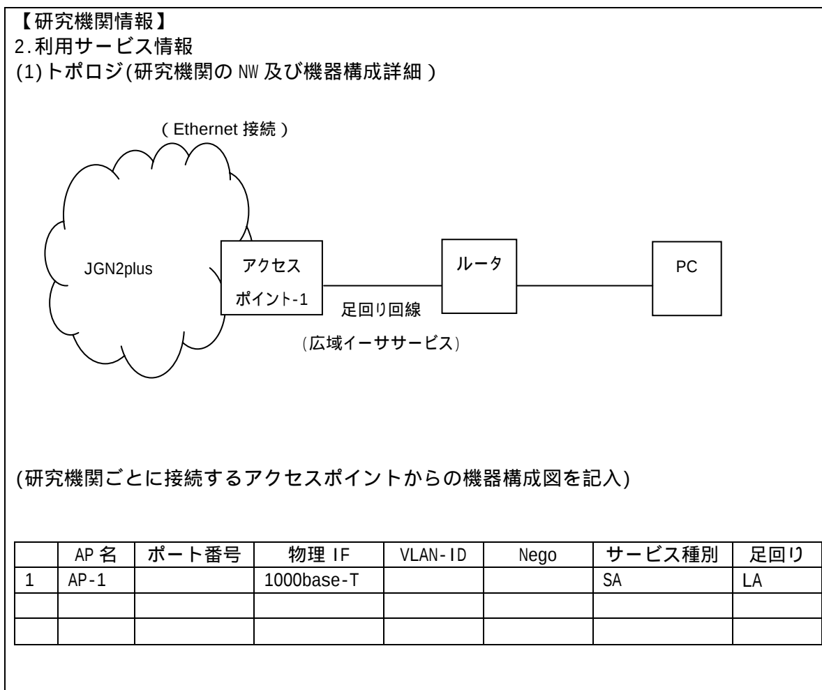
図 3-2 トポロジ図イメージと記載例
